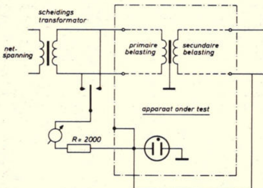
Fig. 6. Met dit VDE 0804 test circuit wordt de lekstroom gemeten, die mogelijk is door een persoon zou vloeien wanneer een condensator in de voeding kortsluit en het chassis per ongeluk wordt aangeraakt.
